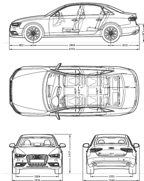
124 Abmessungen Audi A4 Limousine
